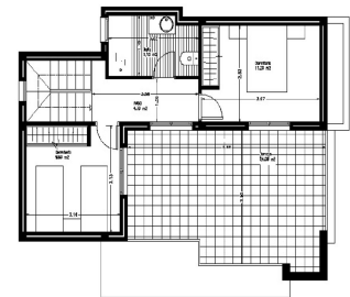
PLANTA ALTA
