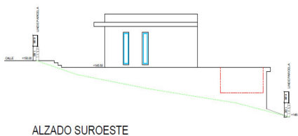
ALZADO SUROESTE
