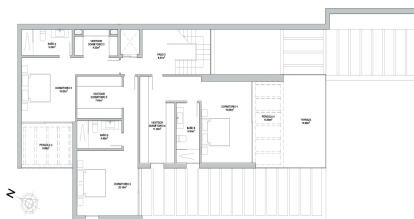
Planta Primera - Zona de noche
