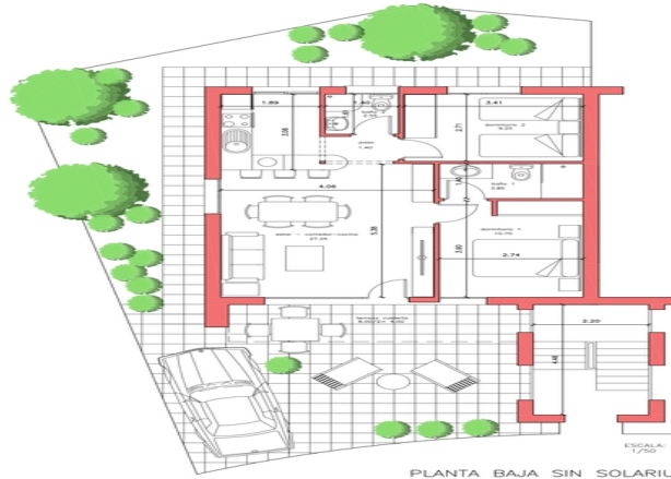
PLANTA BAJA SIN SOLARIUM VIVIENDA 054 SUP. PARCELA= 151,90 M2.
