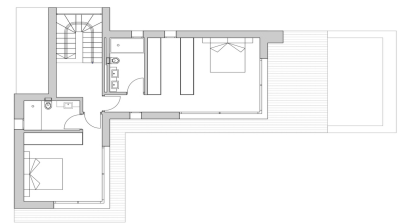
PLANTA ALTA
